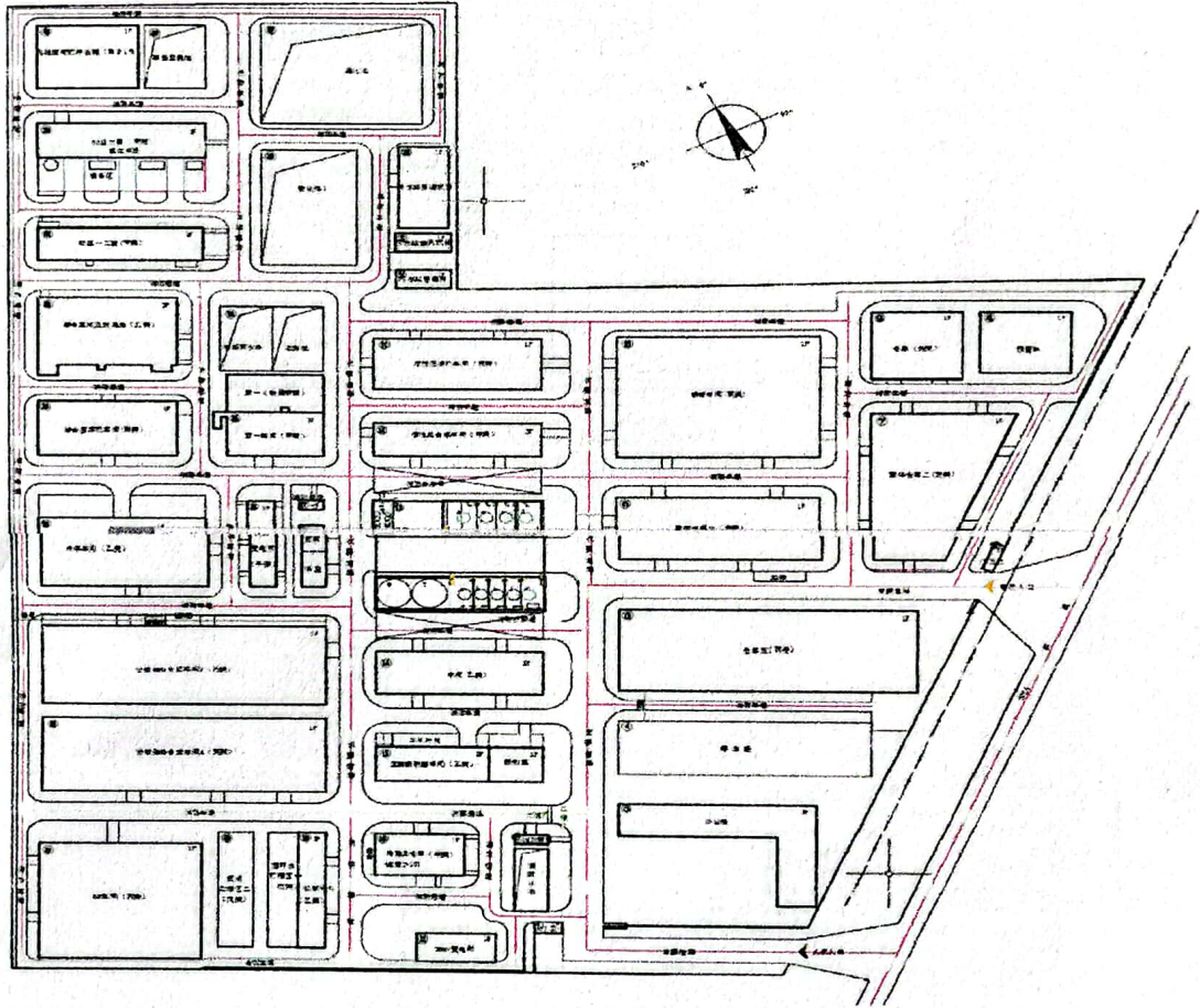
江苏远征化工有限公司老厂区平面布置图
